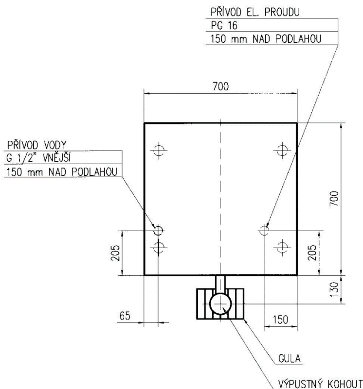
INSTALAČNÍ SCHEMA EL. KOTLE 85 I E-B 85/700
